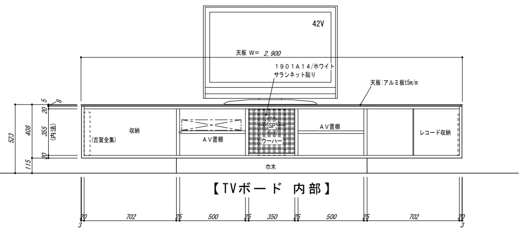
【立面図(閉鎖時)】
