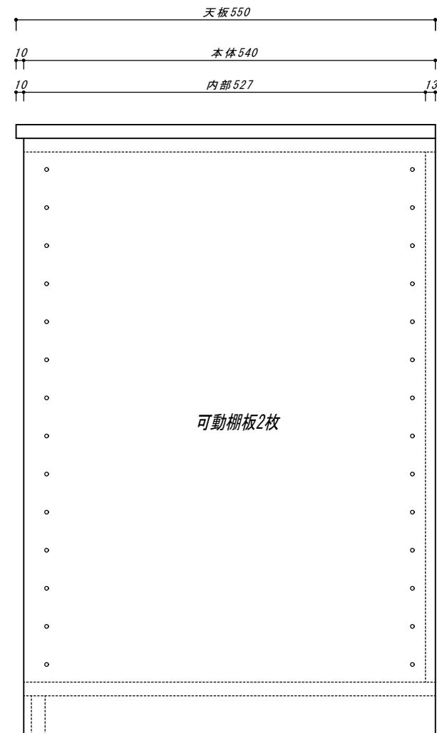
【側面図】
