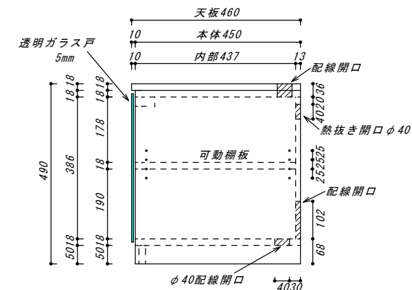
【ガラス両開き戸側横断面図】
