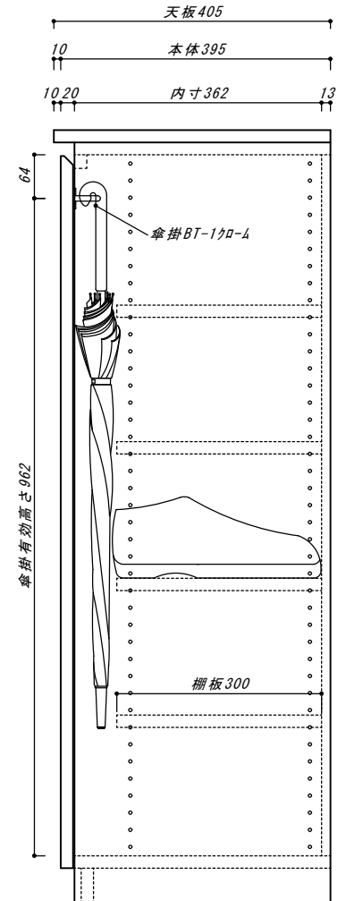
【右側側面図図】
