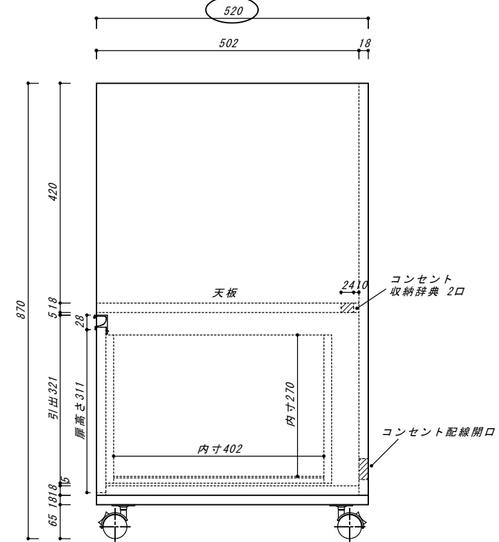
【側面図】
